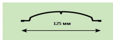
Полукруглый профиль 125 мм
